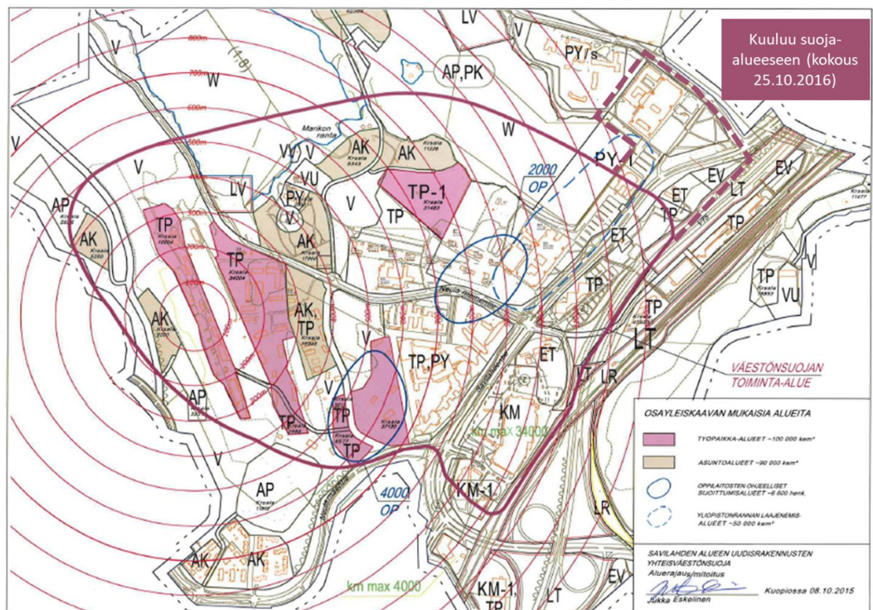
Kuva 1. Suojan toiminta-alue
