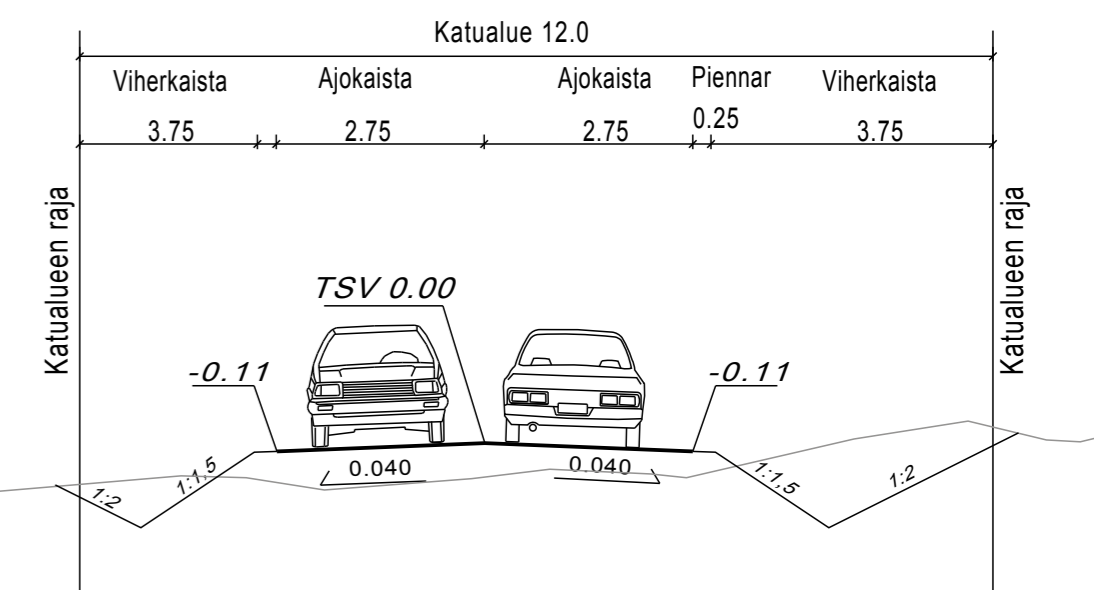
Tyyppipoikkileikkaus A-A 1:100
