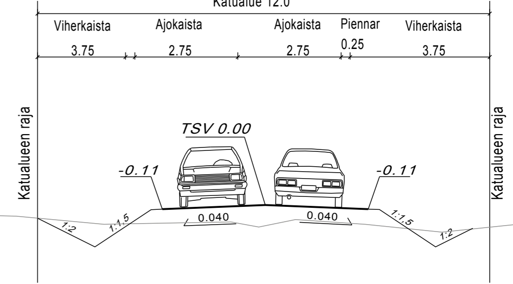
Tyypipoikkileikkaus B-B 1:100 Katualue 12.0
