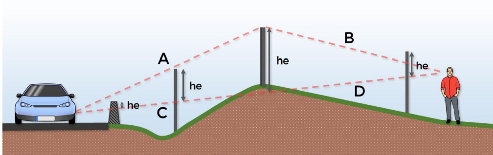
Kuva 8. Melusteen sijainti ja tehollinen korkeus (he) vaikuttavat esteellä saavutettavaan vaimennukseen. Pohjoismaisen tieliikennemelun laskentamallin mukaan estevaimennus on sitä suurempi mitä suurempi on äänilähteestä esteen harjan kautta vastaanottopisteeseen kulkevan etäisyyden ja äänilähteen ja vastaanottopisteen välisen suoran etäisyyden erotus (A+B) - (C+D). Alkuperäinen kuva lähteestä Liikennevirasto 2010.
