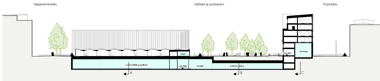
Alueleikkaus 3-3, 1:400
