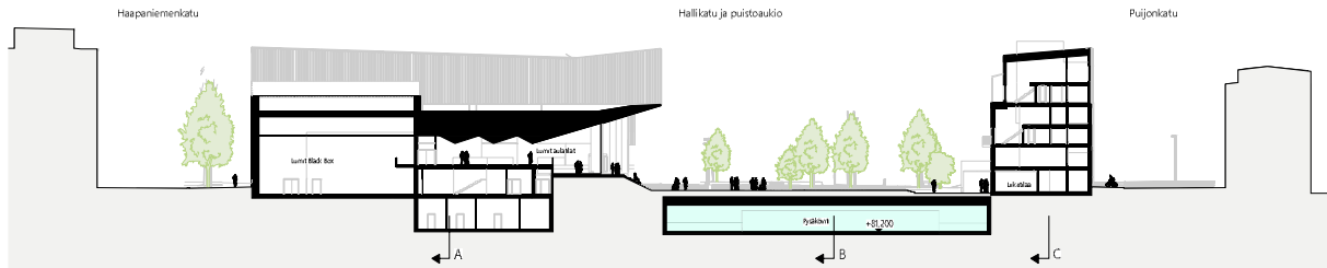
Alueleikkaus 2-2, 1:400
