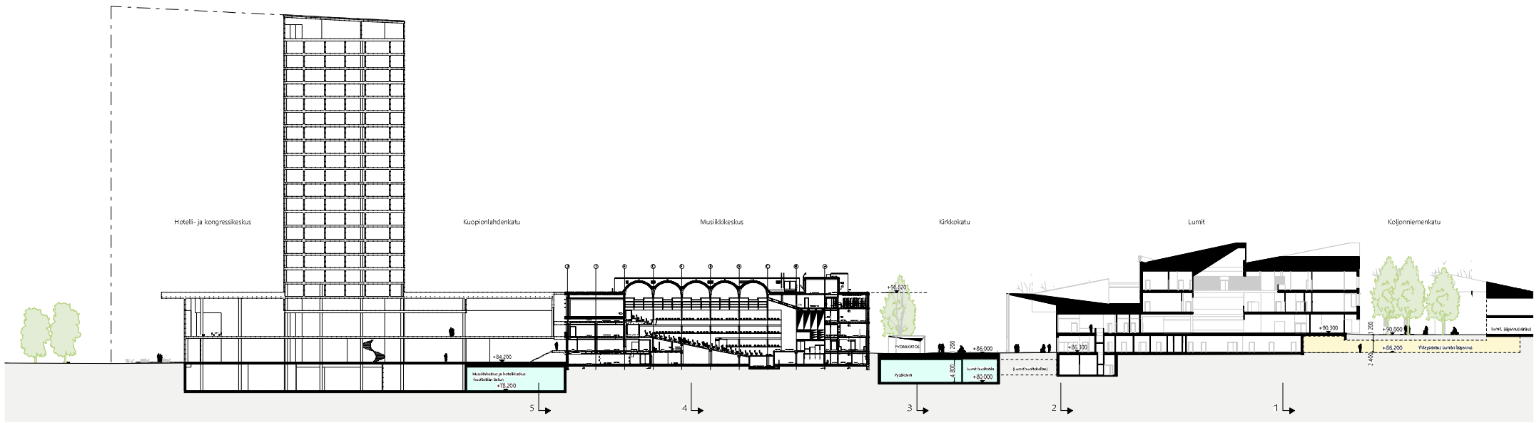
Alueleikkaus A-A, 1:400
