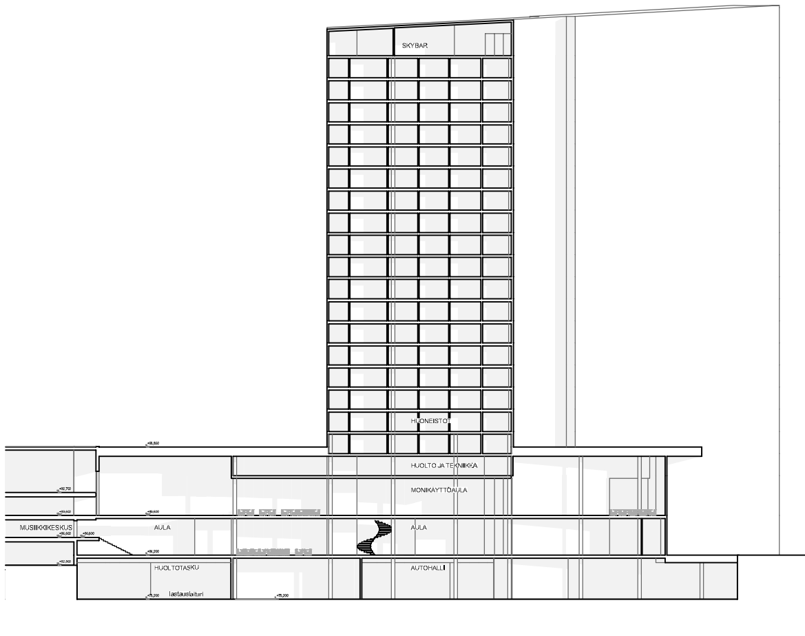
A Leikkaus
