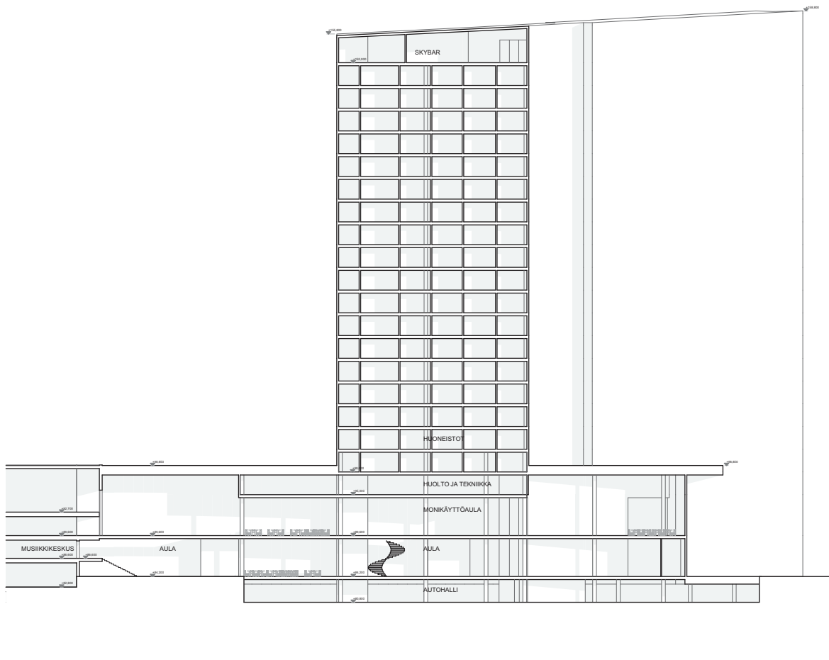
A Leikkaus
