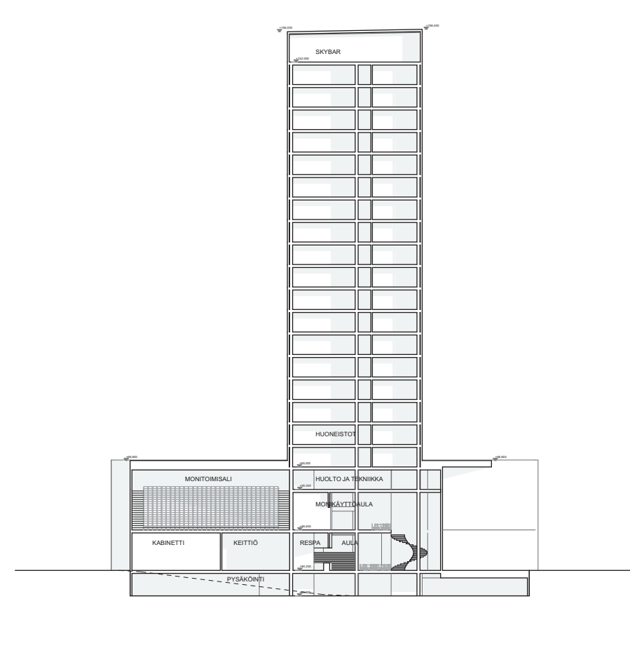
B Leikkaus
