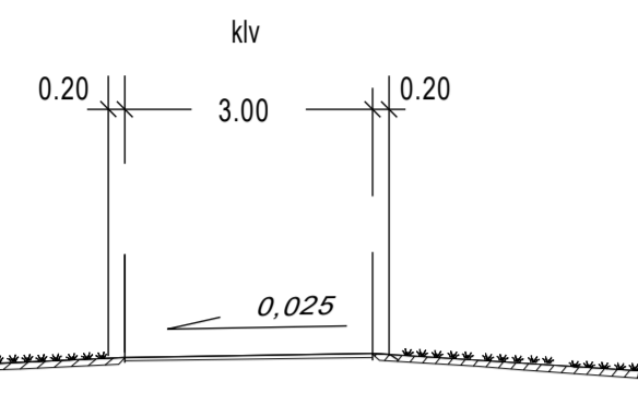
Tyypipoikkileikkaus G-G
