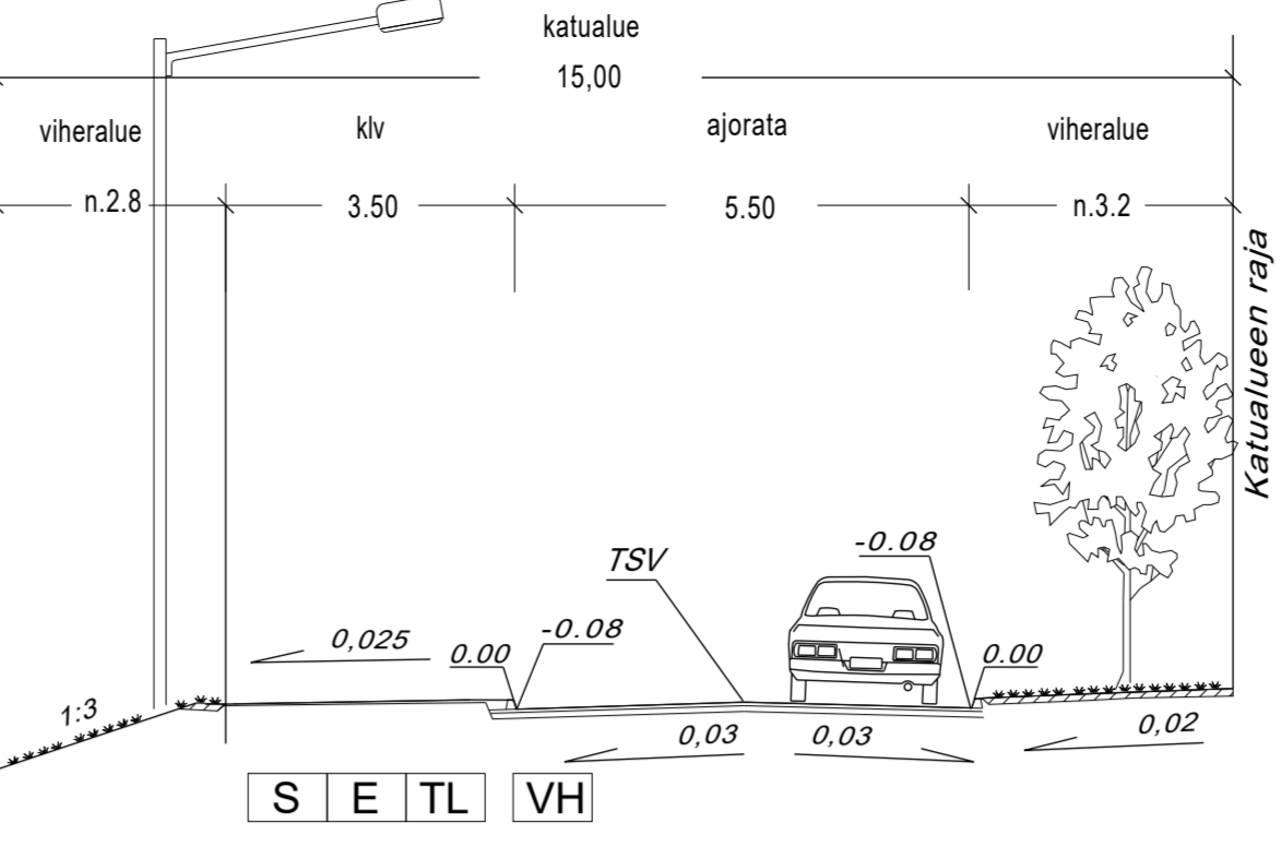
Tyypipoikkileikkaus D-D
