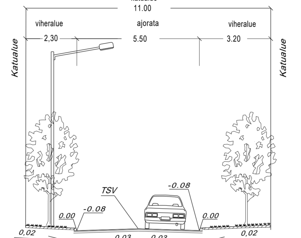
Tyypipoikkileikkaus C-C
