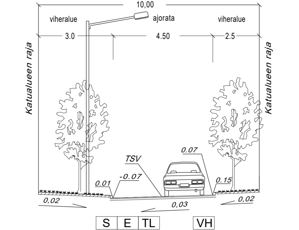
Tyypipoikkileikkaus C-C
