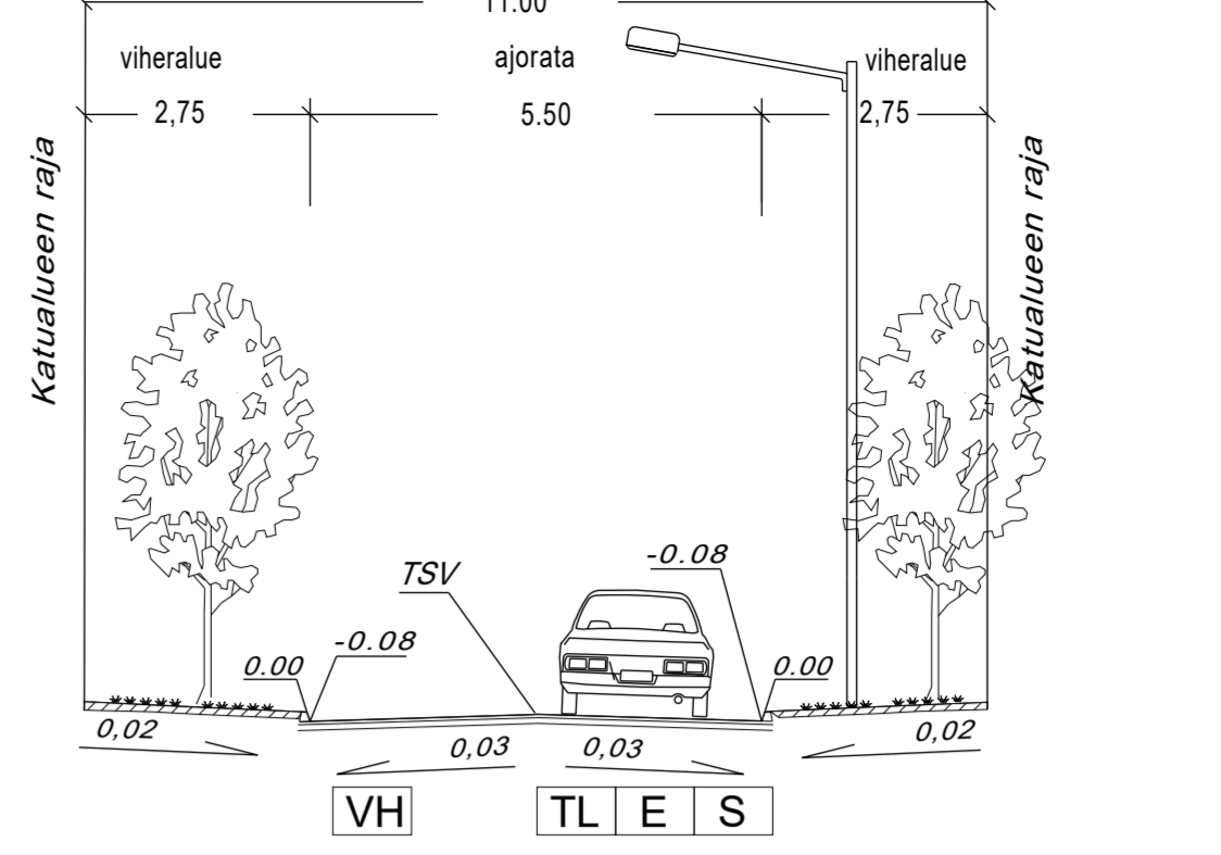
Tyypipoikkileikkaus F-F
