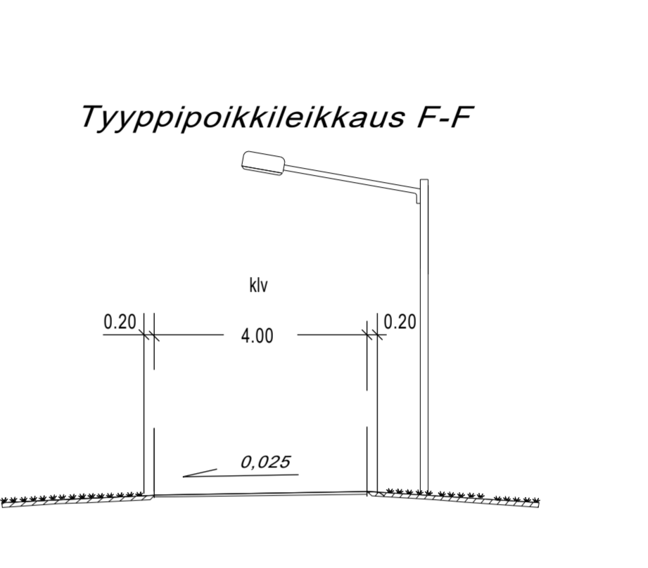
Tyypipoikkileikkaus F-F
