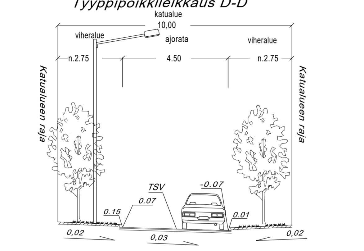
Tyypipoikkileikkaus D-D
