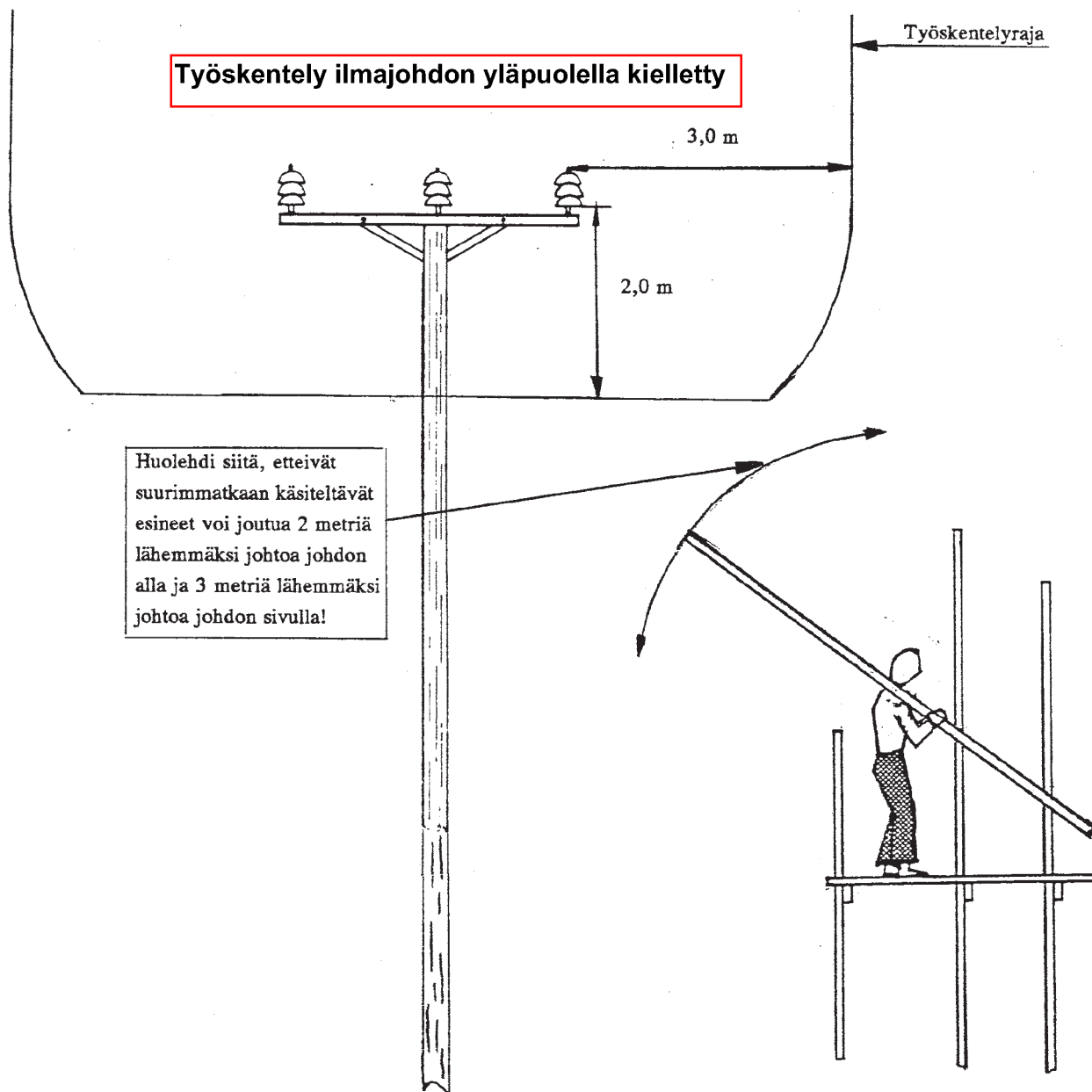
Kuva 10. Vähimmäisetäisyydet 20 kV avojohdon lähellä työskenneltäessä
