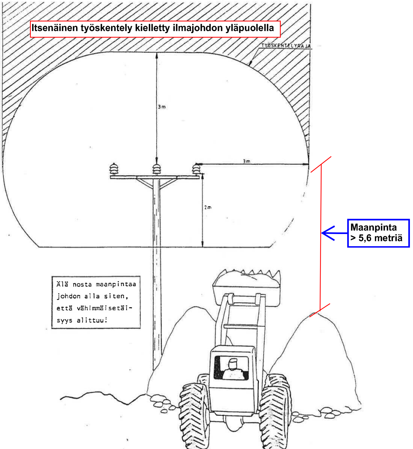
Kuva 12. Vähimmäisetäisyydet työskenneltäessä 20 kV avojohdon läheisyydessä kaivinkoneella, puominosturilla tms. Viivoitetulla alueella sallitaan vain lyhytaikainen työskentely sähkölaitoksen edustajan valvonnassa
