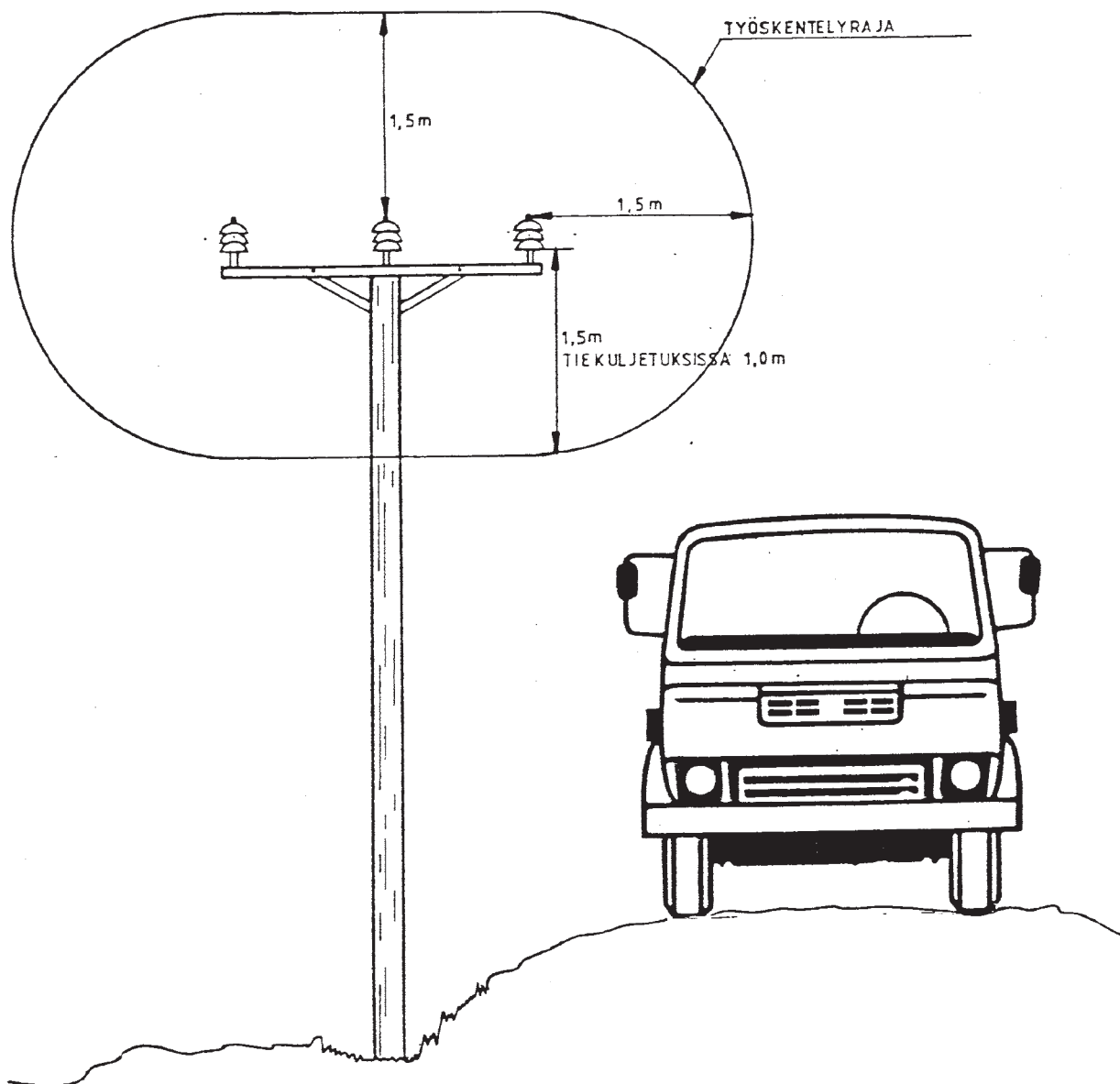
Kuva 11. Vähimmäisetäisyydet 20 kV avojohdosta kuljetuksissa sekä työskenneltäessä koneella, jonka ulottuma ei riipu käyttäjästä.
