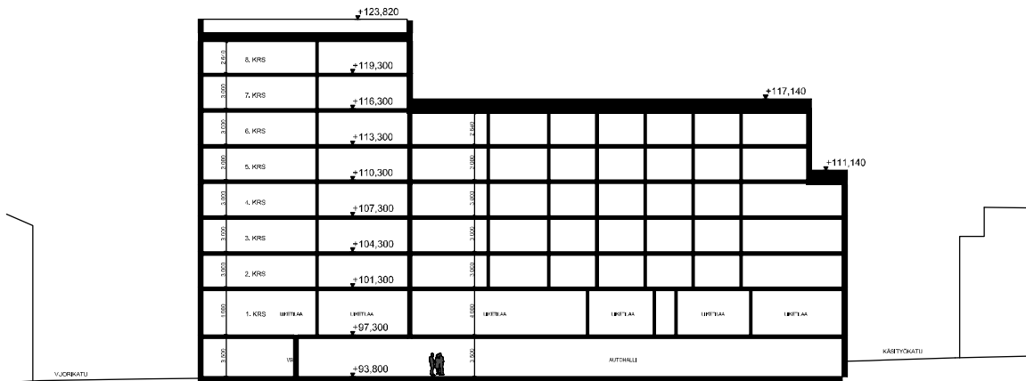
Leikkaus b-b 1:400
