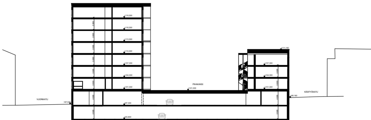
Leikkaus C-C 1:400
