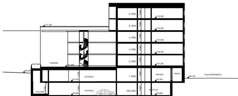
Leikkaus A-A 1:400
