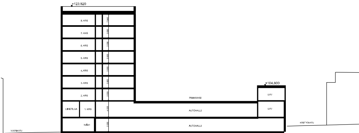
Leikkaus c-c 1:400
