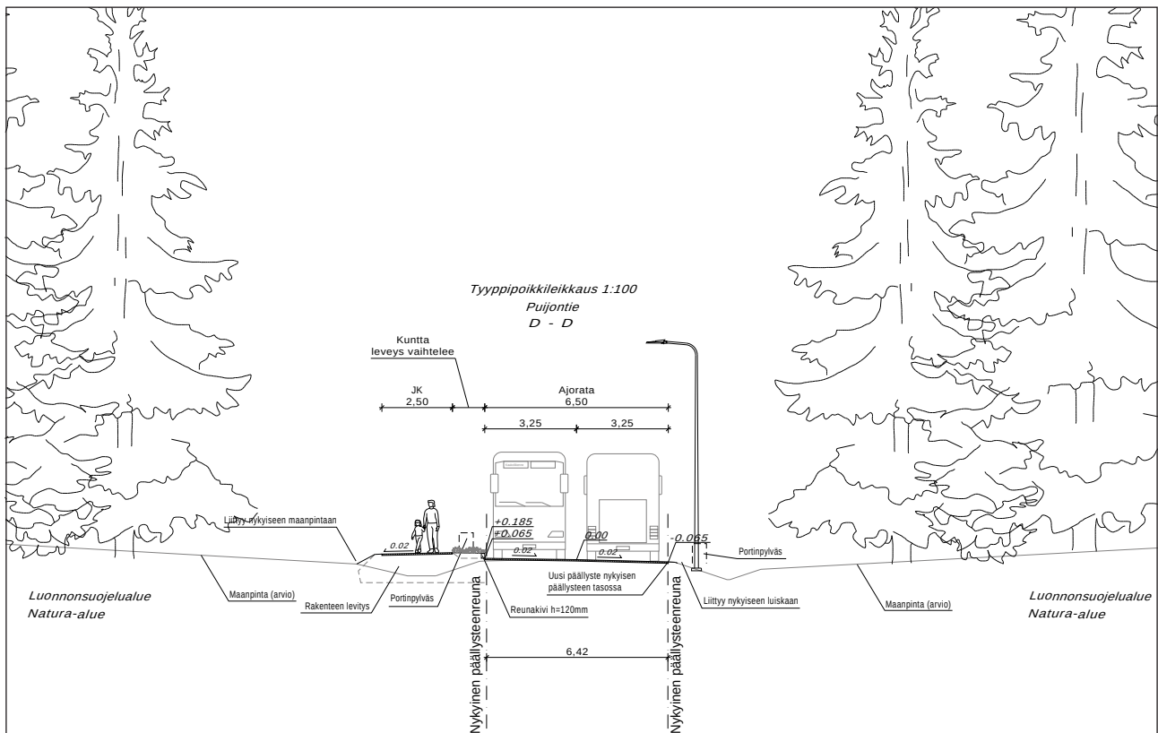
Kuva 63. Puijontien poikkileikkaus yläpäästä.
