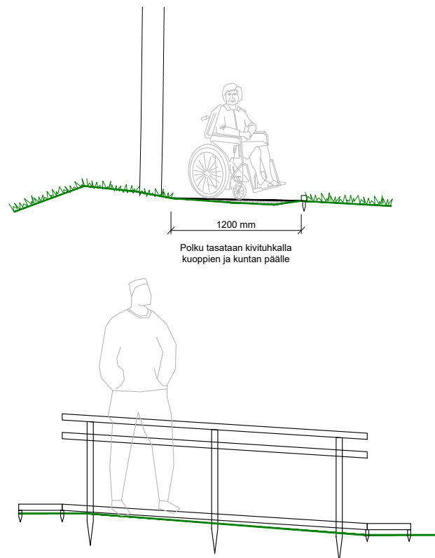
Kuva 70. Eteläisen parannetun luontoreitin periaate ja jyrkkiin kohtiin sijoitettava kaide.
