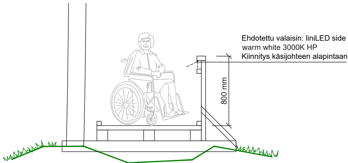
Kuva 65. Maan päälle asetettavan kansirakenteen periaate.
