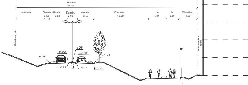
Tyyppiokileikkaus Sarastuskaari B-B
