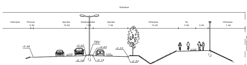
Tyyppiokileikkaus Sarastuskaari A-A
