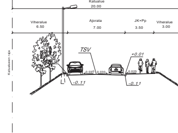
Tyyppiokileikkaus Loistekatu E-E
