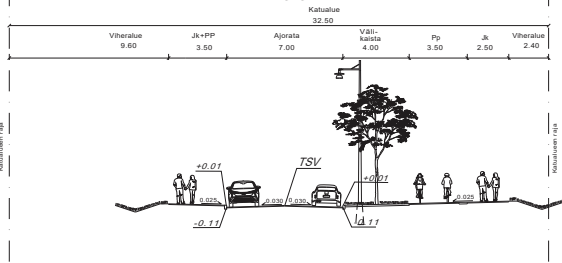
Tyyppiokileikkaus Sarastuskaari C-C
