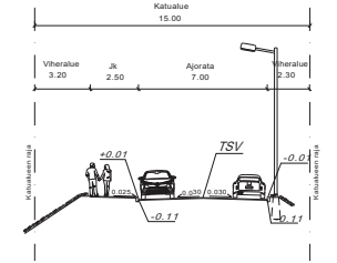
Tyyppiokileikkaus Sädekuja F-F
