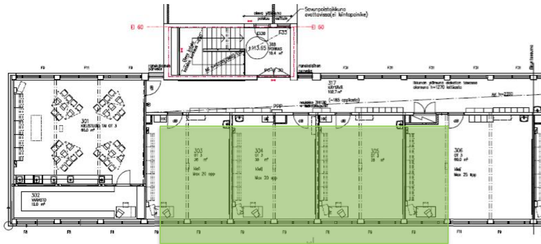
Kuva 3 Pääkoulu 3. kerroksen opetustilat, jotka palautetaan alkuperäiseen luokkakokoon kahdeksi opetustilaksi.
