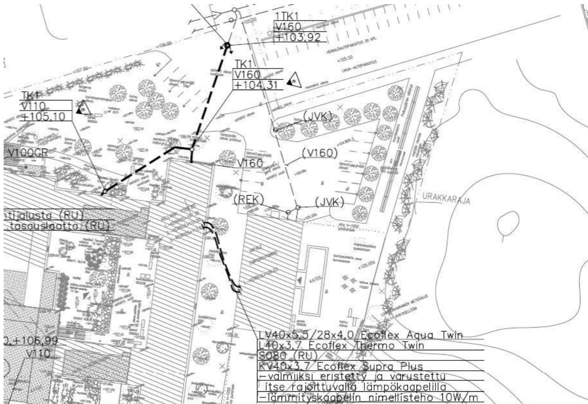
Kuva 6 Nykyiset talotekniset liittymät peruskorjauksen 2006 mukaisesti. Huom! korot eivät vastaa nykyistä korkojärjestelmää.
