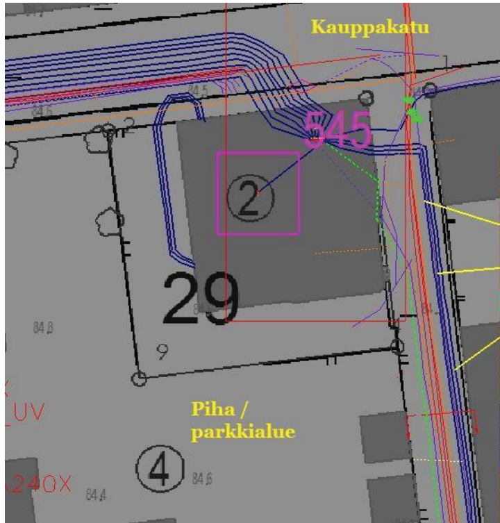
Kuva 2.2. Sähköaseman maanalaiset kaapeloinnit pihaan ja katuun nähden.
